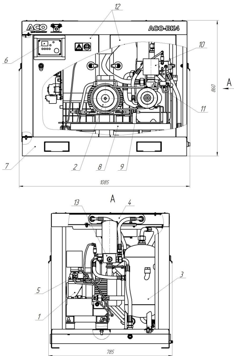
Рисунок 2. Агрегат компрессорный.
